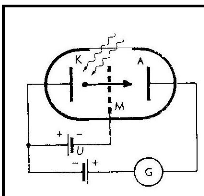
Obr. 1. 4: Schéma experimentu ke studiu fotoelektrického jevu.
