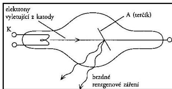
Obr. 1. 3. Schéma rentgenky.
