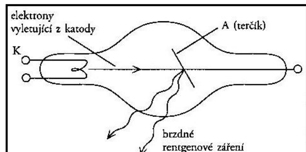
Obr. 1. 5: Schéma rentgenky.
